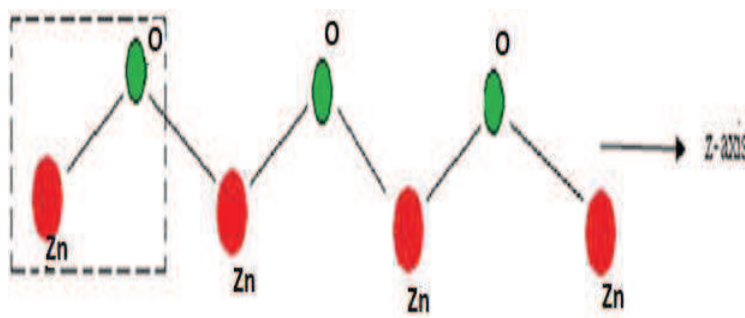
(b) 2-atom Zigzag Nanowire
